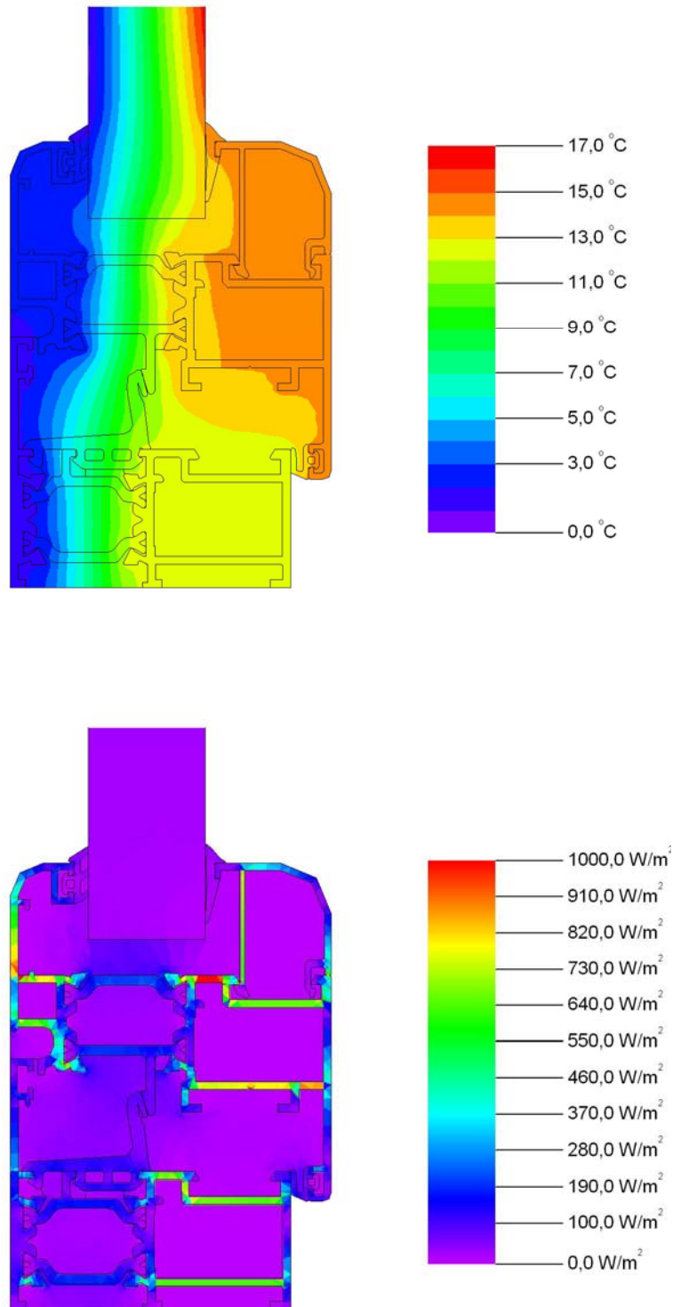
Fig. 6. Andamento delle temperature e dei flussi di calore nel nodo 02
