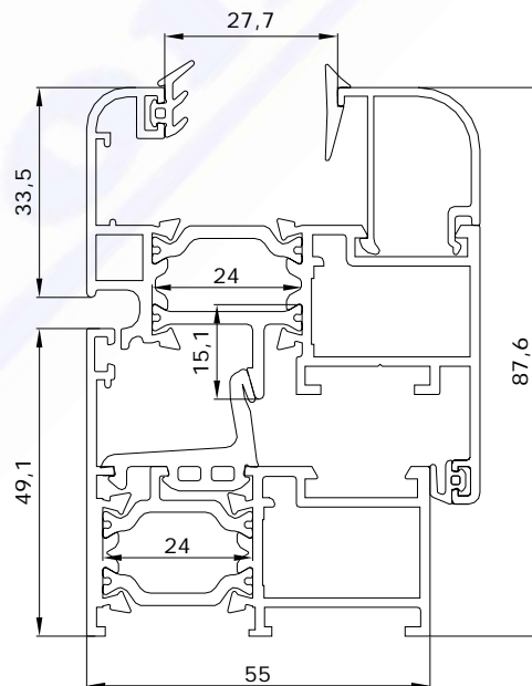
Fig. 3: Sezione del nodo 02 (nodo laterale) del campione analizzato
