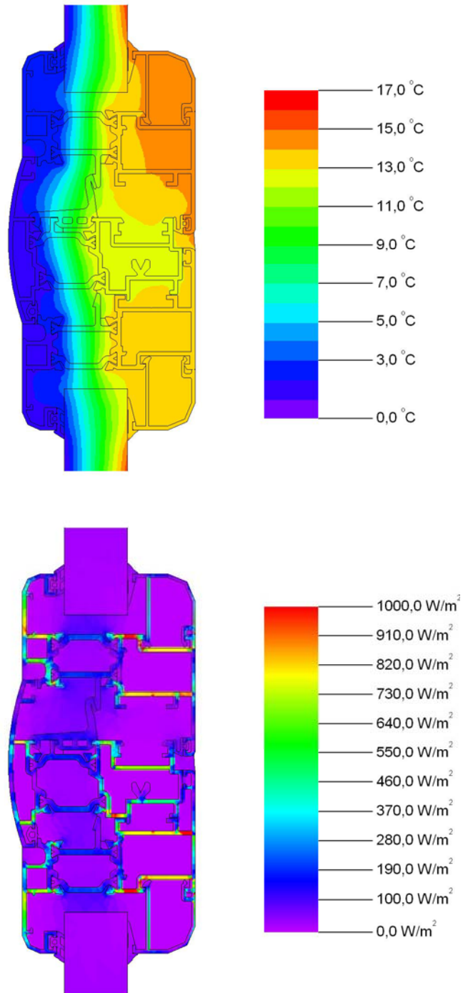
Fig. 5. Andamento delle temperature e dei flussi di calore nel nodo 01
