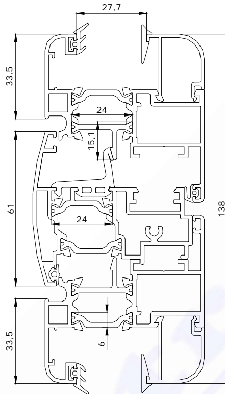
Fig. 2: Sezione del nodo 1 (nodo centrale) del campione analizzato
